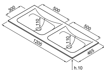
VIVO 120 2M dupla mosdó
