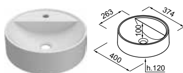
PURO T ROUND pultra ültethető mosdó 76 200,-
