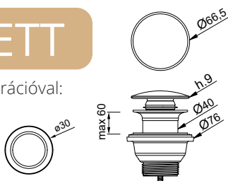
LEFOLYÓ SZETT, FEHÉR klikk-klakk +túlfolyó karika
